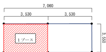
■テント仕様
